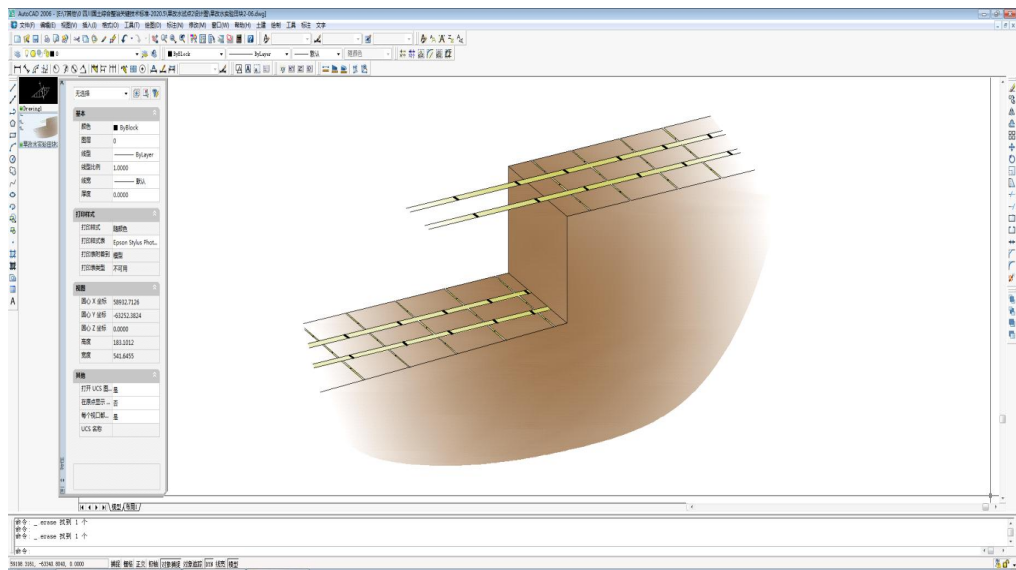
图 E.2 竹筋田坎示意图
