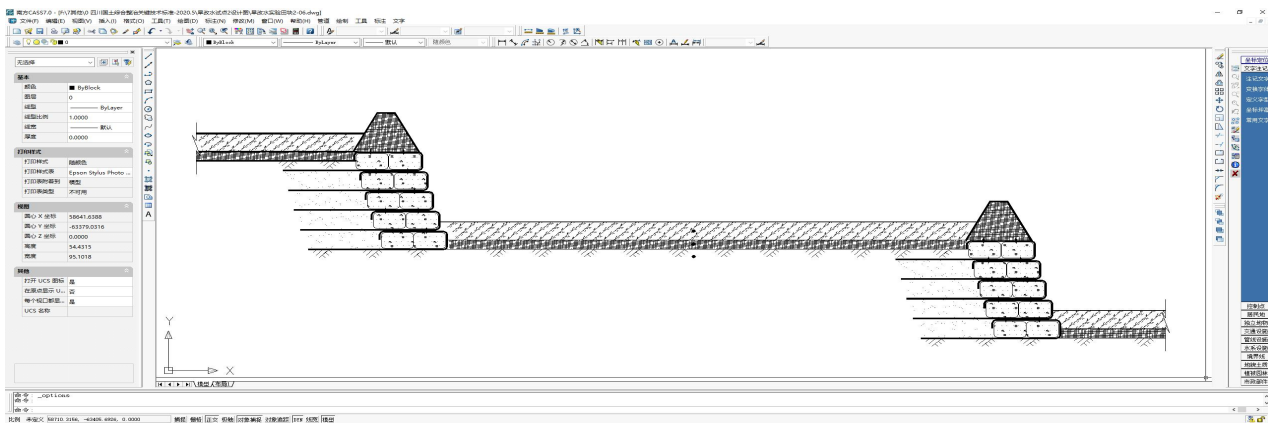
图 E.1 单向土工格栅加筋土生态田坎示意图
